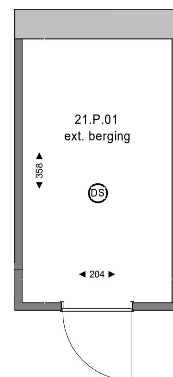
plattegrond berging 1 : 50 4e verdieping
