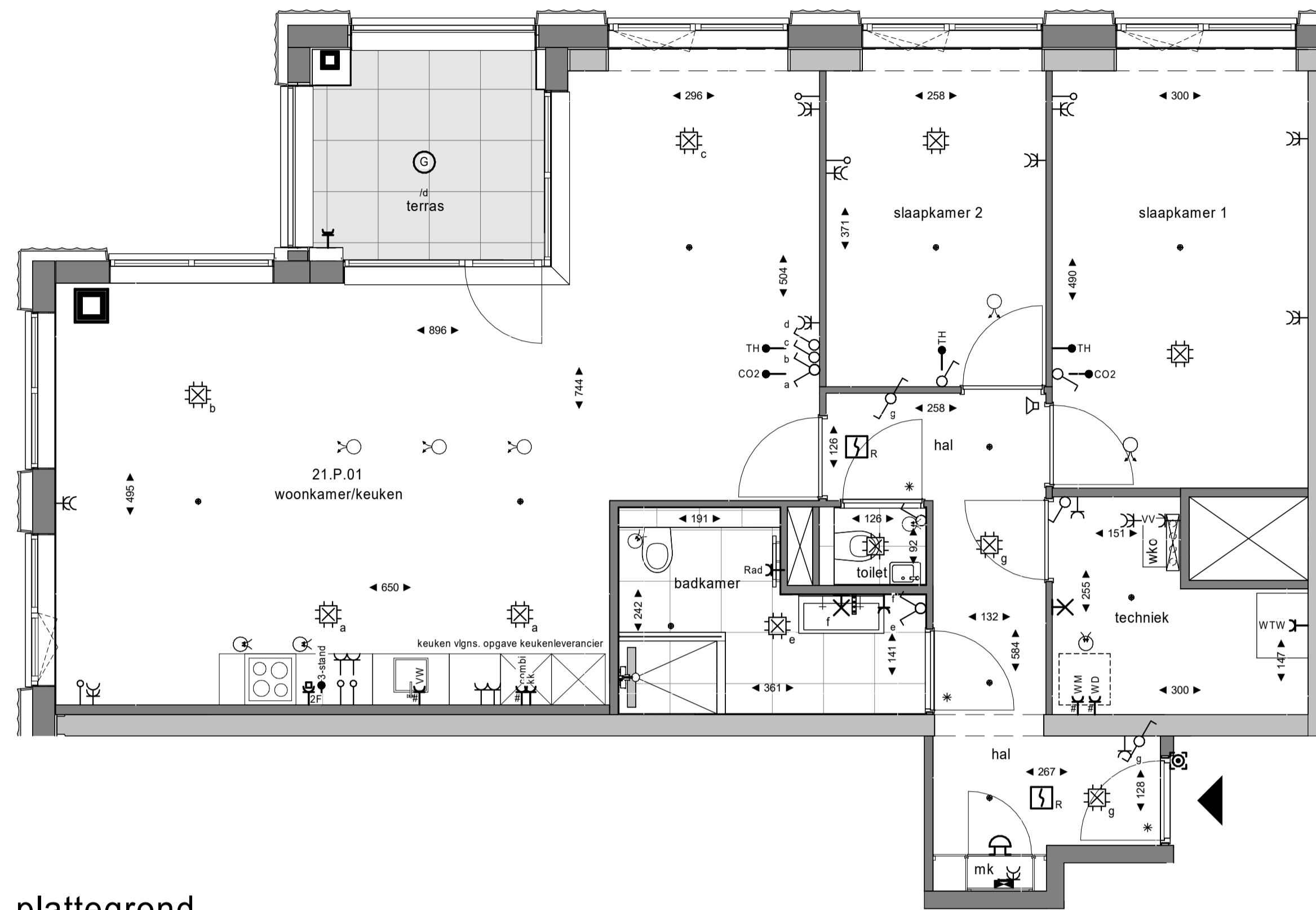
plattegrond 1 : 50 21e verdieping
